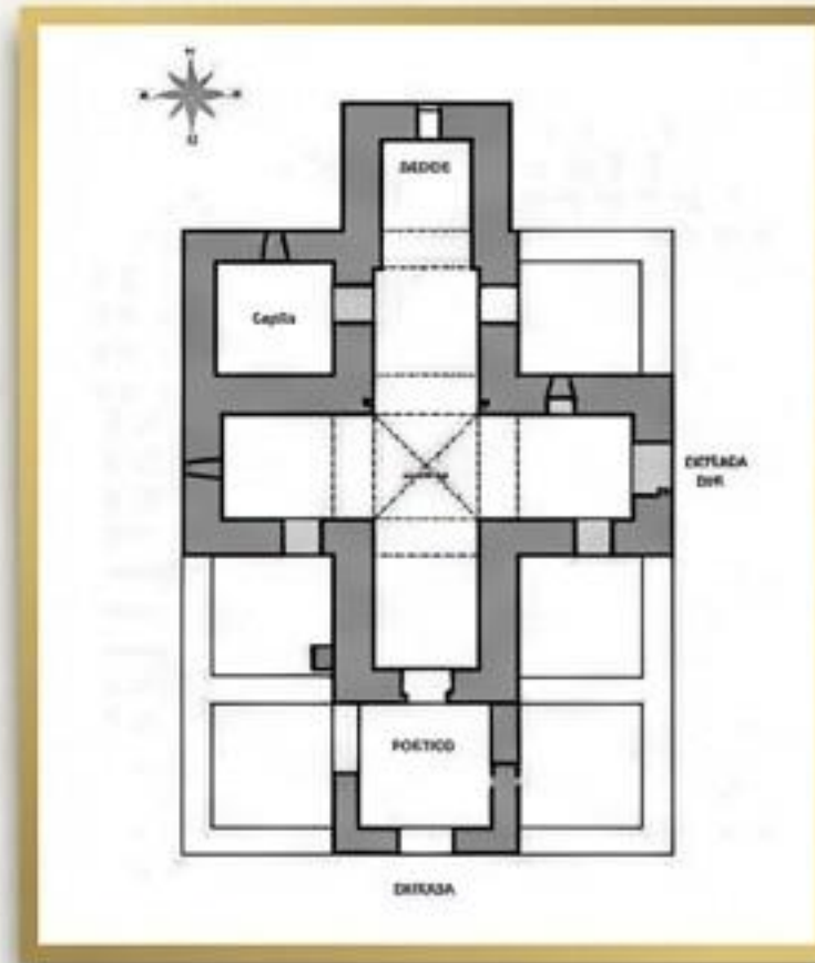
CRUCIFORME Santa Comba de Bande
