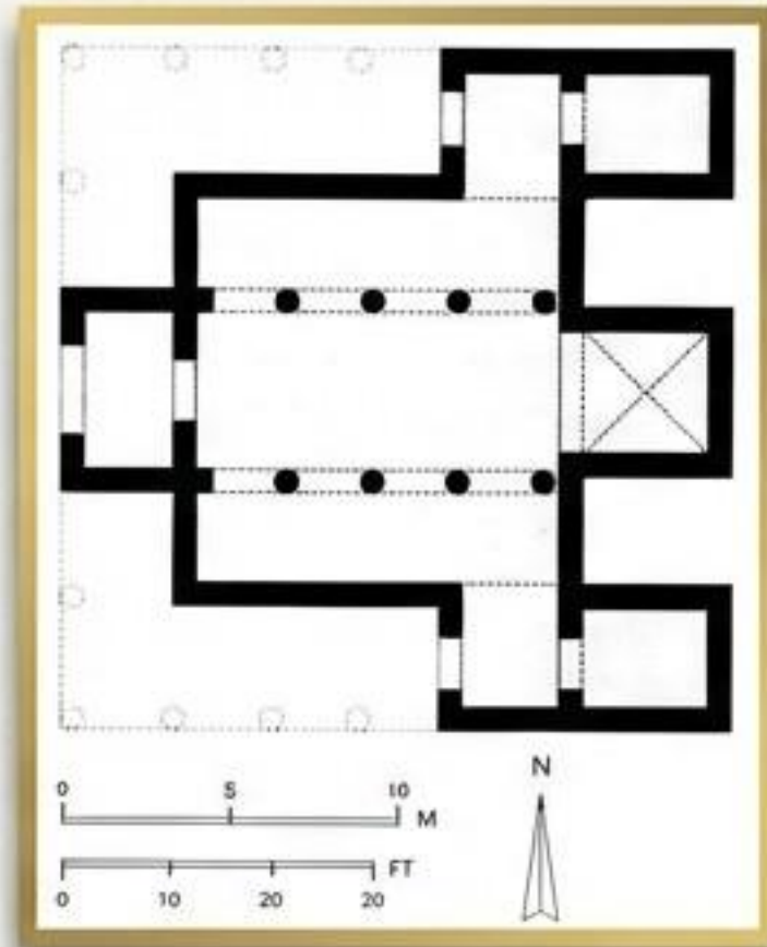
BASILICAL San Juan de Baños
